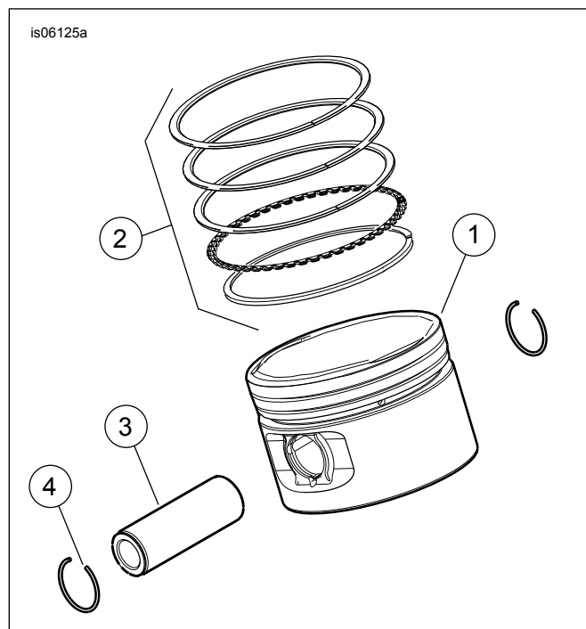
Figur 4. Reservedele: Sæt med forreste og bageste stempel
