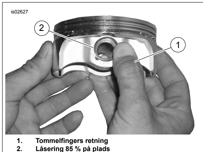
Figur 3. Monter låseringsklips (standardstempel vist)
