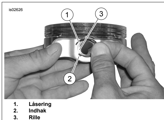
Figur 2. Låseringsklips og stempel (standardstempel vist)
