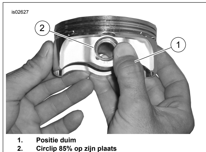
Afbeelding 3. Circlip installeren (algemene zuiger getoond)
