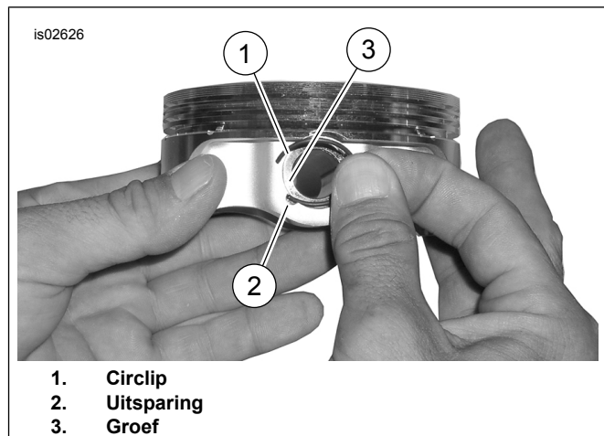
Afbeelding 2. Circlip en Zuiger (algemene zuiger getoond)
