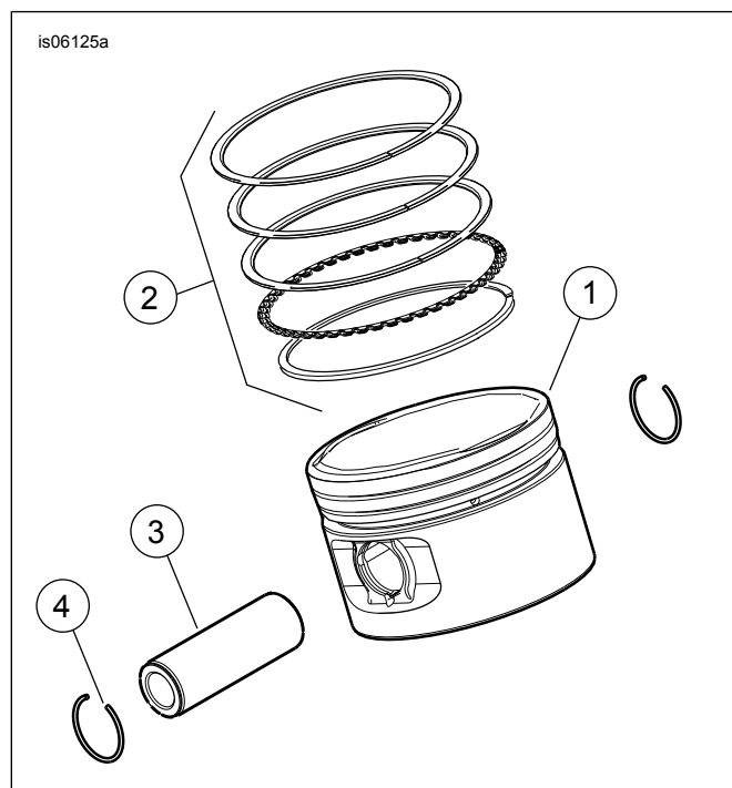
Afbeelding 4. Serviceonderdelen: Voorste en achterste zuigersets
