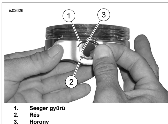
Ábra 2. Seeger gyűrű és dugattyú (általános dugattyú látható)
