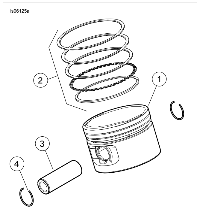
Ábra 4. Szervizelhető alkatrészek: Első és hátsó dugattyú készletek
