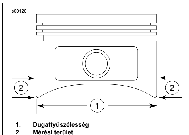
Ábra 1. Dugattyú mérések
