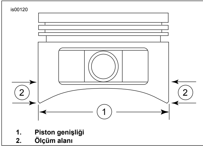
Şekil 1. Piston Ölçümleri
