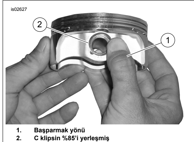
Şekil 3. C Klipsi Takma (genel piston gösterilmiştir)
