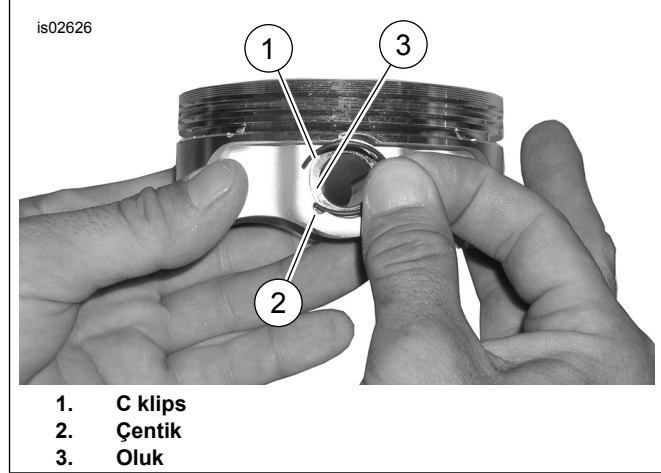
Şekil 2. C klips ve Piston (genel piston gösterilmiştir)
