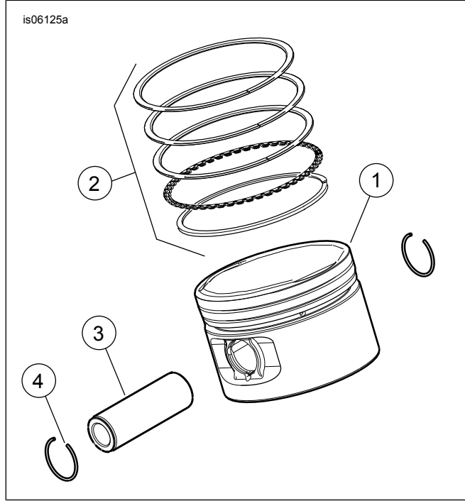
Şekil 4. Servis Parçaları: Ön ve Arka Piston Kitleri
