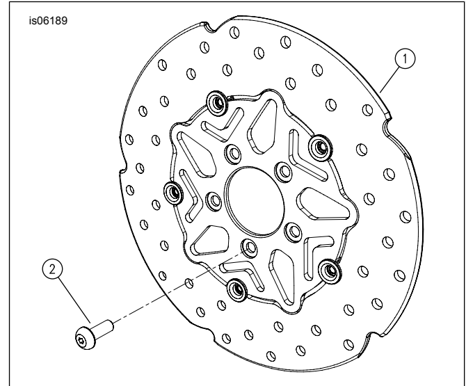
Figure 1. Pièces de rechange : Kits de rotor de frein avant flottant (disque)
