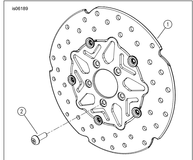
Figura 1. Parti di ricambio: Kit disco del freno flottante anteriore
