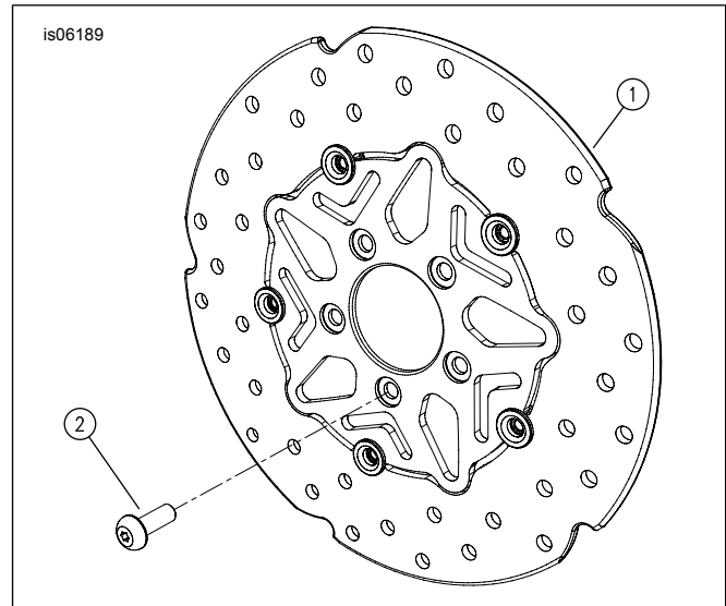
Abbildung 1. Ersatzteile: Schwimmend gelagerte Hinterradbremsscheibensätze (angezeigte Stinger-Bauart)
