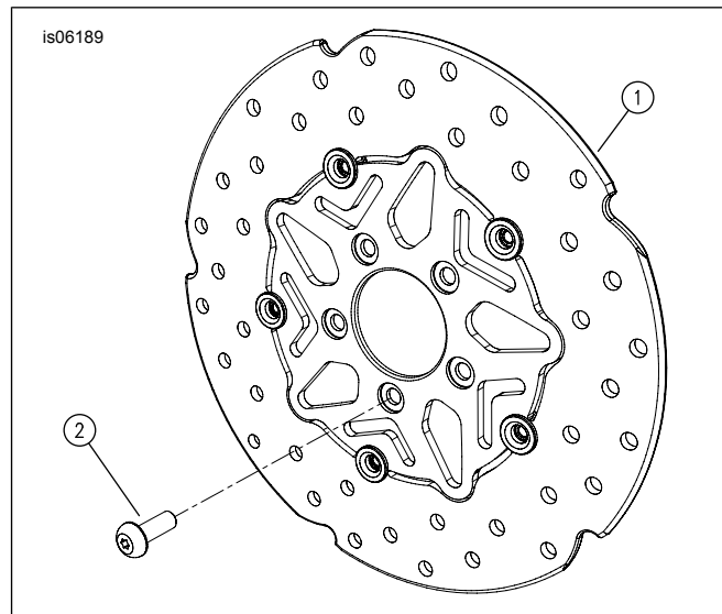
Figura 1. Parti di ricambio: Kit disco del freno flottante posteriore (in figura lo stile Stinger)
