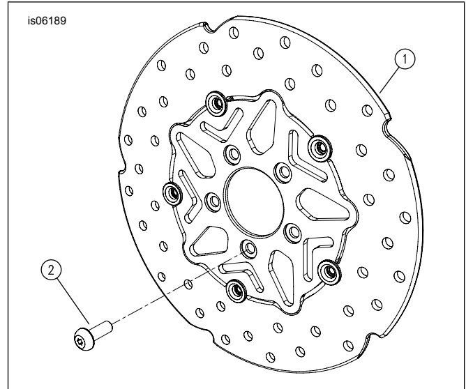
Figura 1. Piezas de servicio: Kits de rotor flotante del freno trasero (disco) (se muestra el estilo para llanta Stinger)
