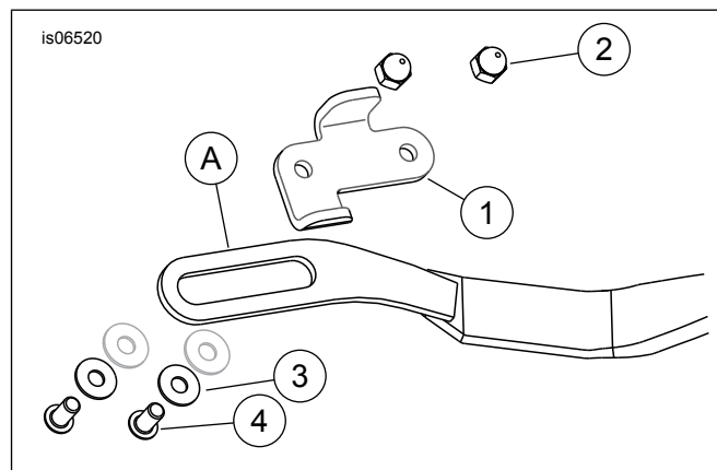
Figura 2. Peças de reposição: Kit de extensão do cavalete lateral (suporte de pé estilo XL mostrado)
