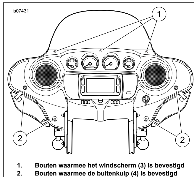
Afbeelding 1. Kuip-/windscherm bouten
