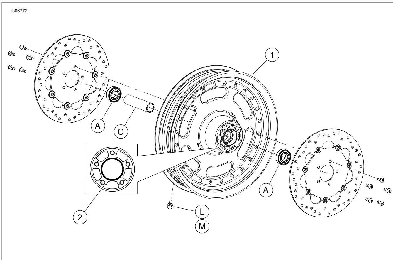
Afbeelding 1. Serviceonderdelen: Cutback voorwiel Fat Bob
