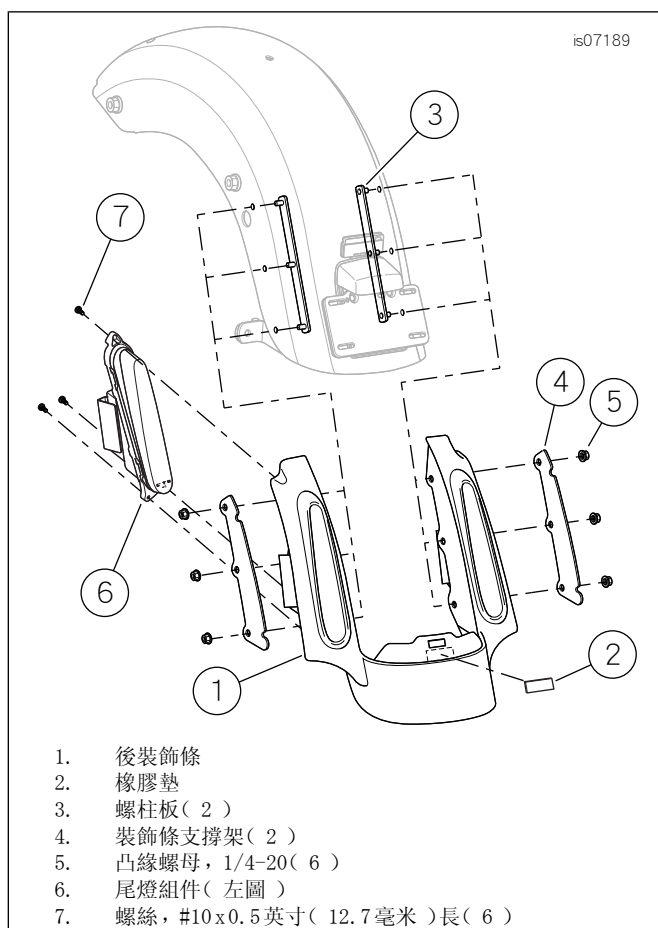
圖4. 後裝飾條安裝
