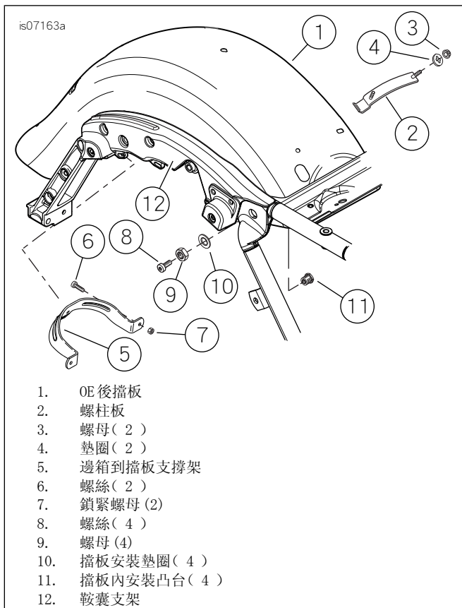
圖1。拆下後擋板物品
