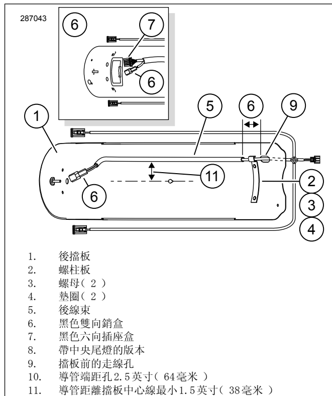
圖2。安裝後擋板線束
