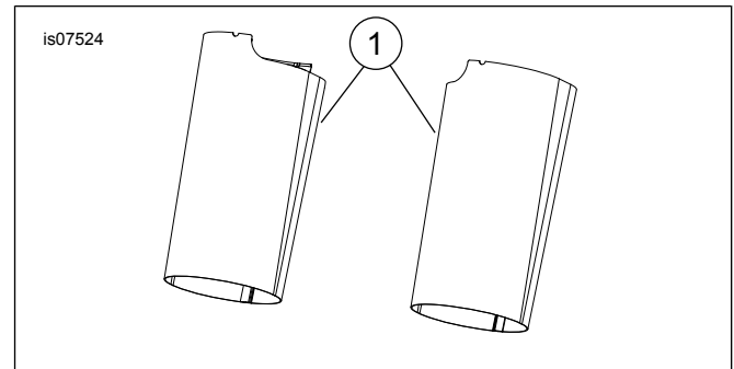
Abbildung 1. Ersatzteile: Gabelgleitrohr-Abdeckungen
