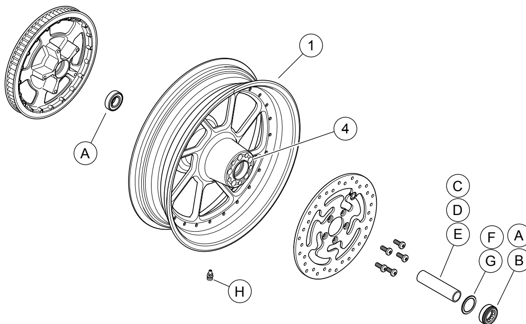
Afbeelding 1. Serviceonderdelen: Road Winder achterwielen
