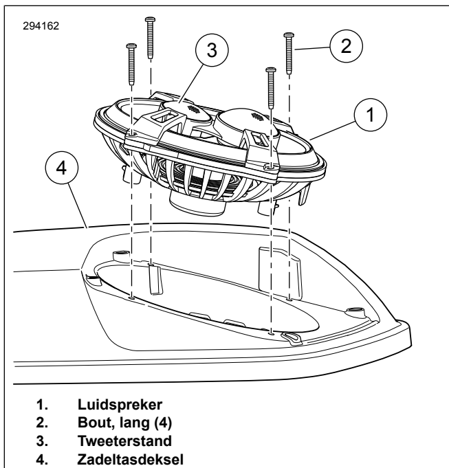
Afbeelding 1. Luidsprekerstand
