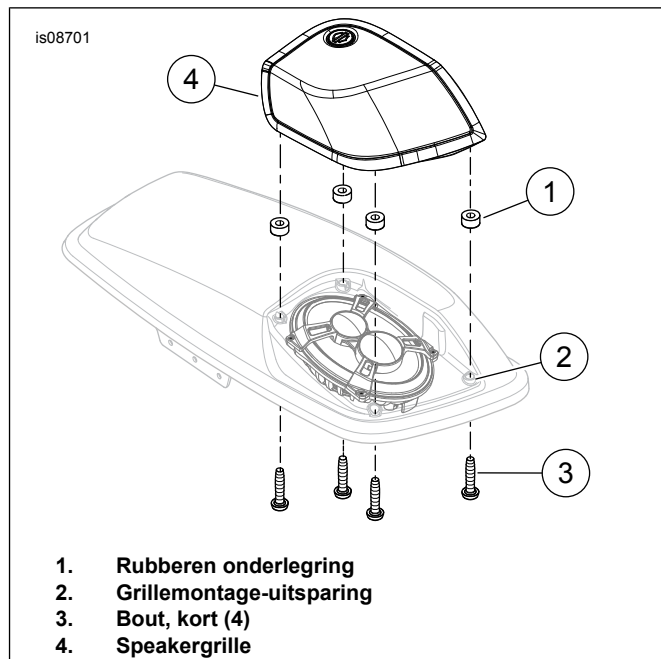
Afbeelding 2. Grillemontage
