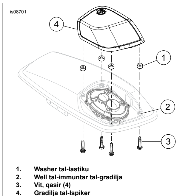
Figura 2. Installazzjoni tal-Gradilja
