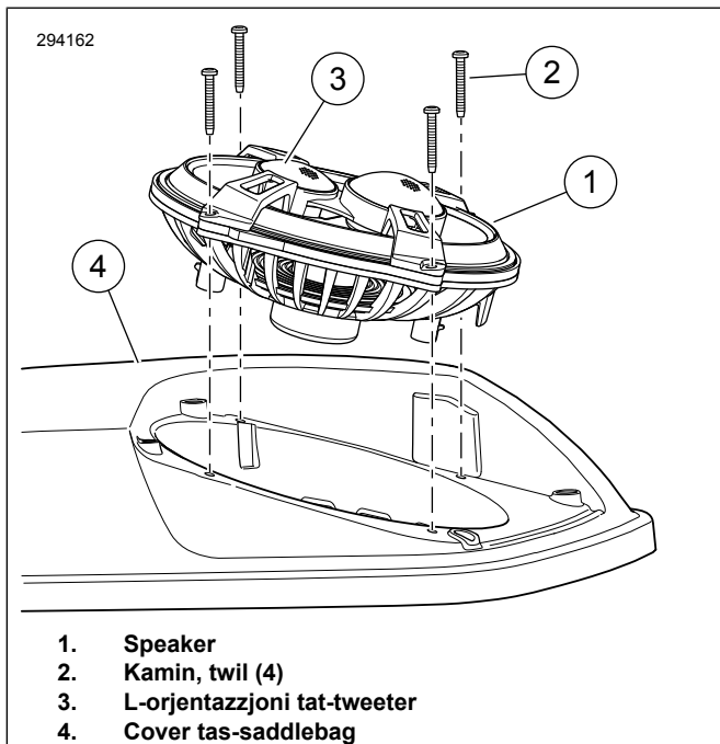
Figura 1. L-orjentazzjoni tal-ispiker
