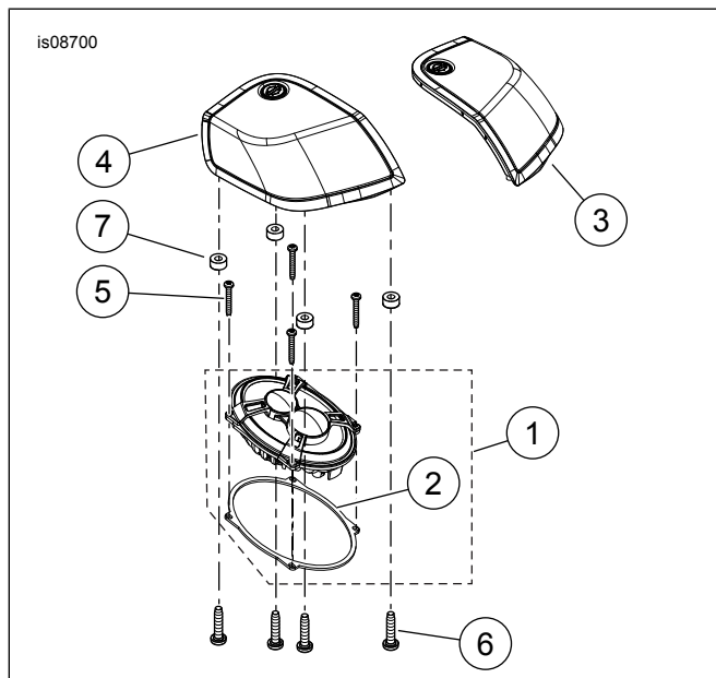
Figur 3. Servicedeler, Boom! Audio Stage II salveskehøyttalersett
