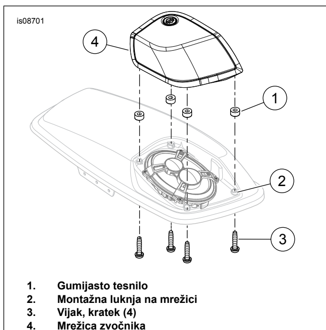
Slika 2. Namestitev mrežice
