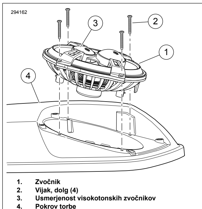
Slika 1. Usmerjenost zvočnikov
