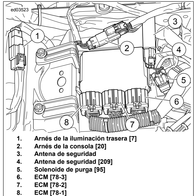
Figura 1. Debajo del asiento: FLHR/C
