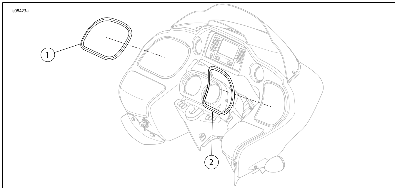
图2。维修零件
