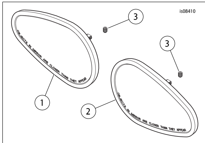
图1。维修零件：挡风玻璃装饰后视镜套件
