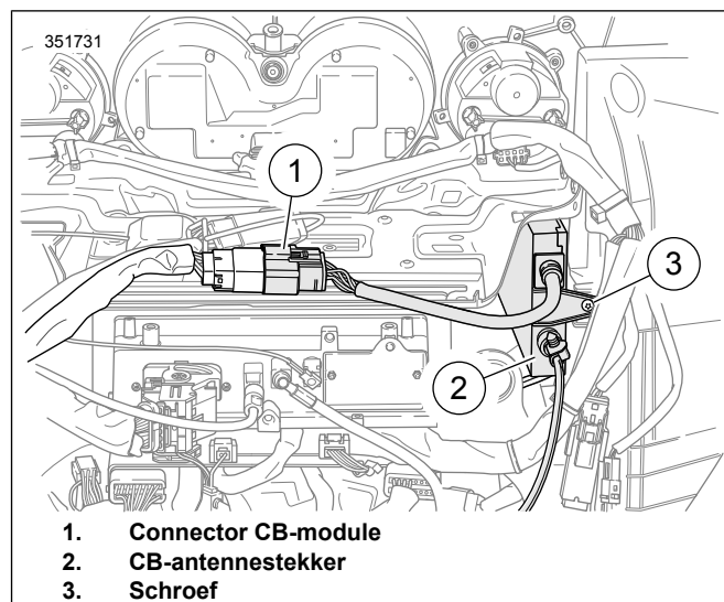
Afbeelding 3. Kabelboomstekkers binnenkuip
