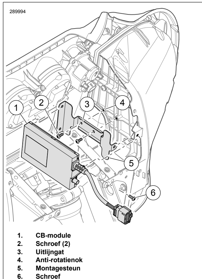
Afbeelding 2. Installeer de CB-module: Op de voorvork gemonteerde kuip
