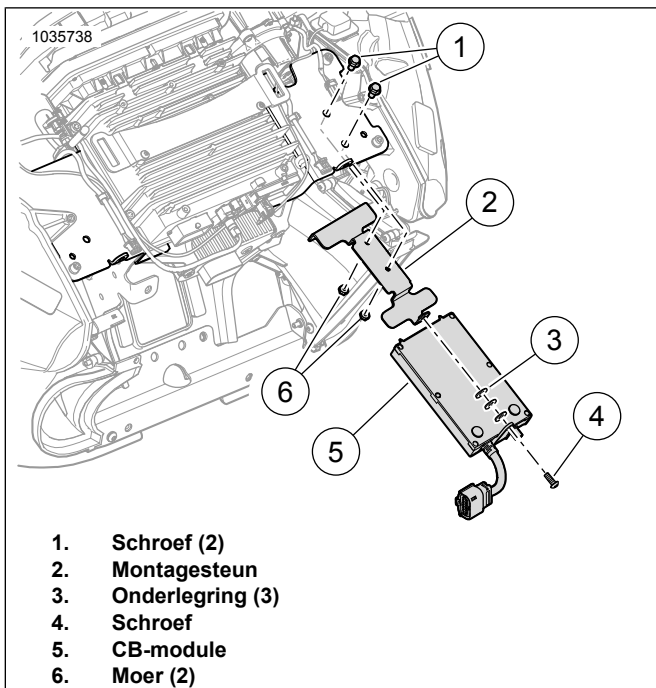
Afbeelding 4. Installeer de CB-module: Op het frame gemonteerde kuip
