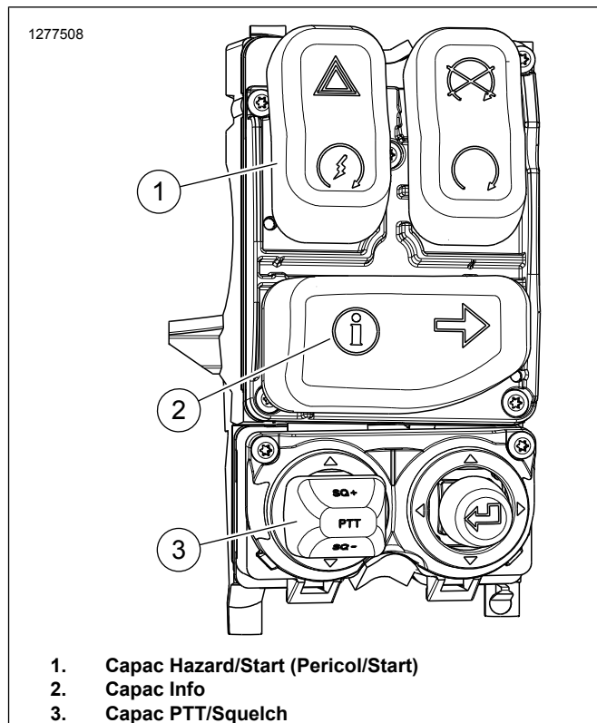
Figura 6. Control dreapta 2014 și ulterioare (71500130C)
