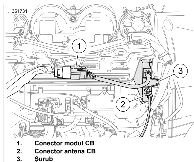
Figura 3. Conectori de cablaj carenaj interior
