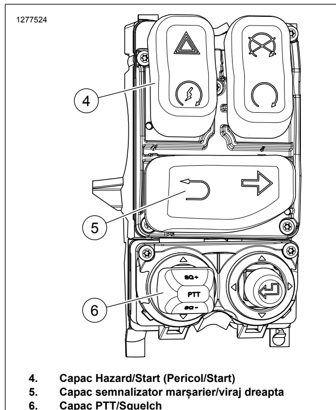
Figura 7. Vedere modul control dreapta modele 2019 și ulterioare după înlocuirea capacului comutatorului
