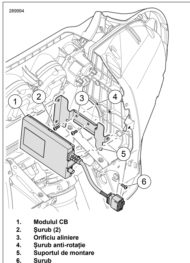
Figura 2. Instalați modulul CB: Carenajul montat pe furcă
