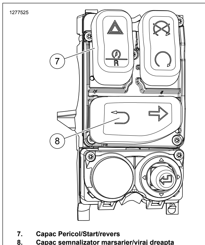
Figura 8. Control dreapta Trike 2019 și ulterioare (OE)
