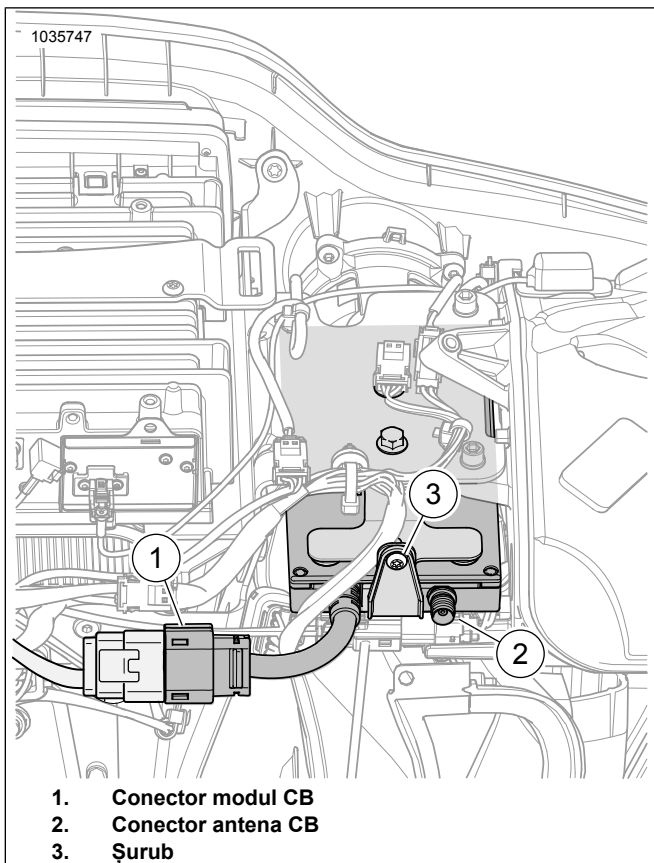
Figura 5. Conectori de cablaj carenaj interior
