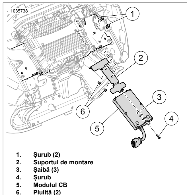
Figura 4. Instalați modulul CB: Carenajul montat pe cadru
