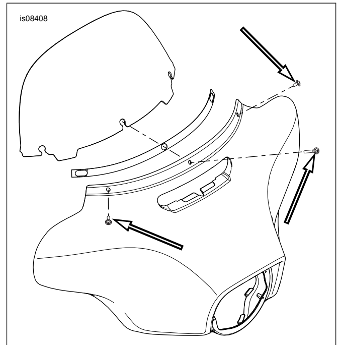
Figura 1. Remova e descarte os parafusos
