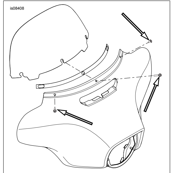
Figura 1. Extracción y desecho de los tornillos
