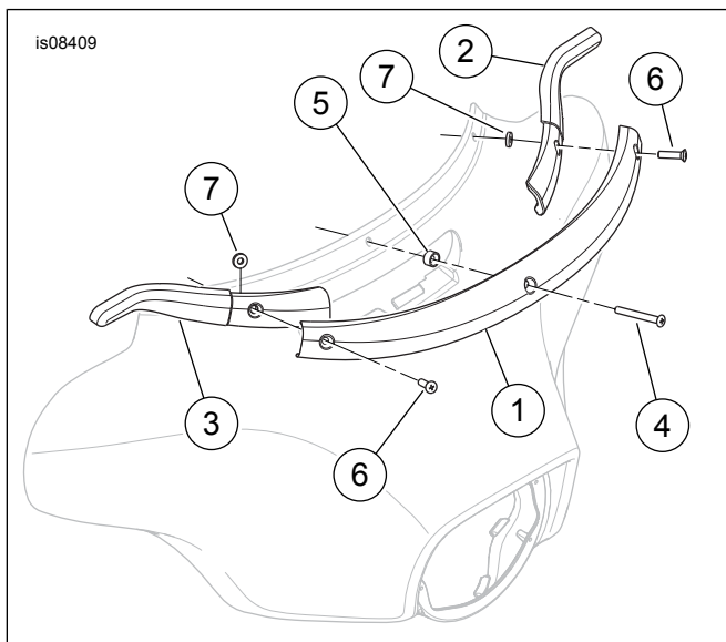
Figura 2. Piezas de servicio: Kit de soportes de espejos decorativos para parabrisas
