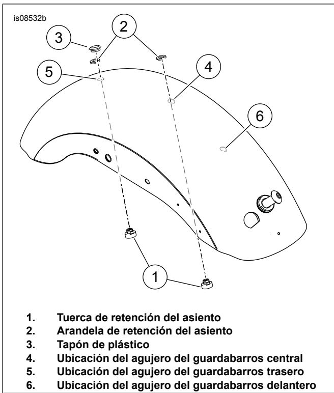
Figura 2. Ubicación de la arandela y la tuerca de retención del asiento
