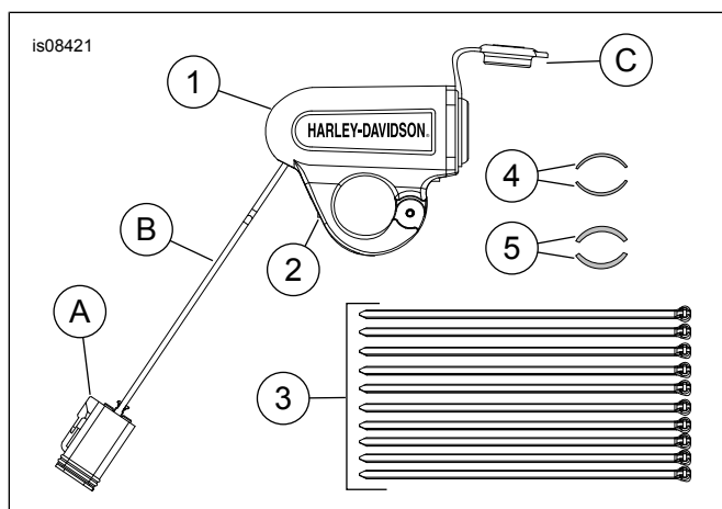
Ilustrace 3. Servisní díly: 12voltový napájecí zdroj řídítek
