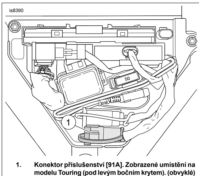
Ilustrace 2. Konektor příslušenství
