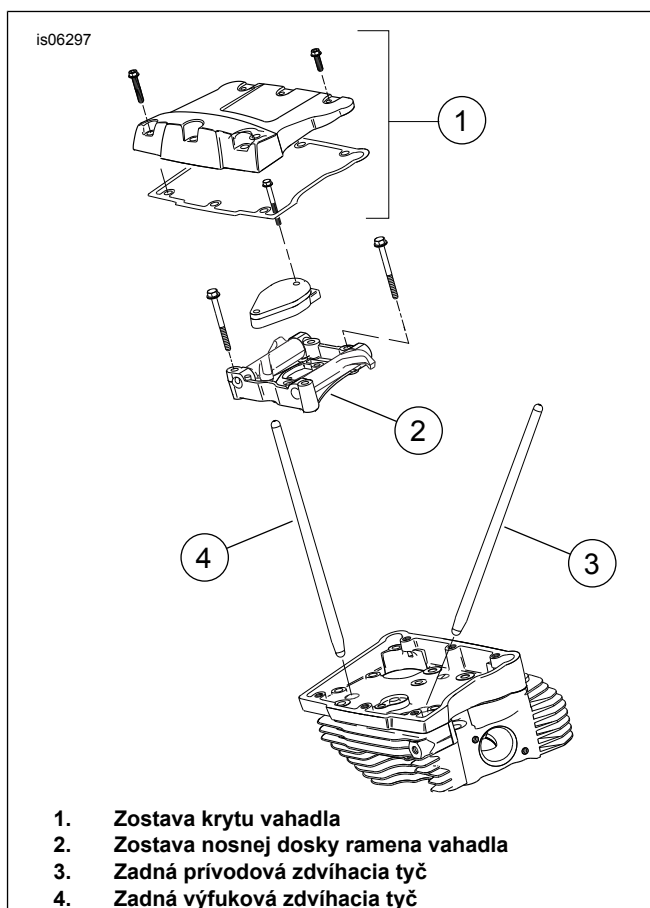
Obrzok 6. Zdvhacie tyy
