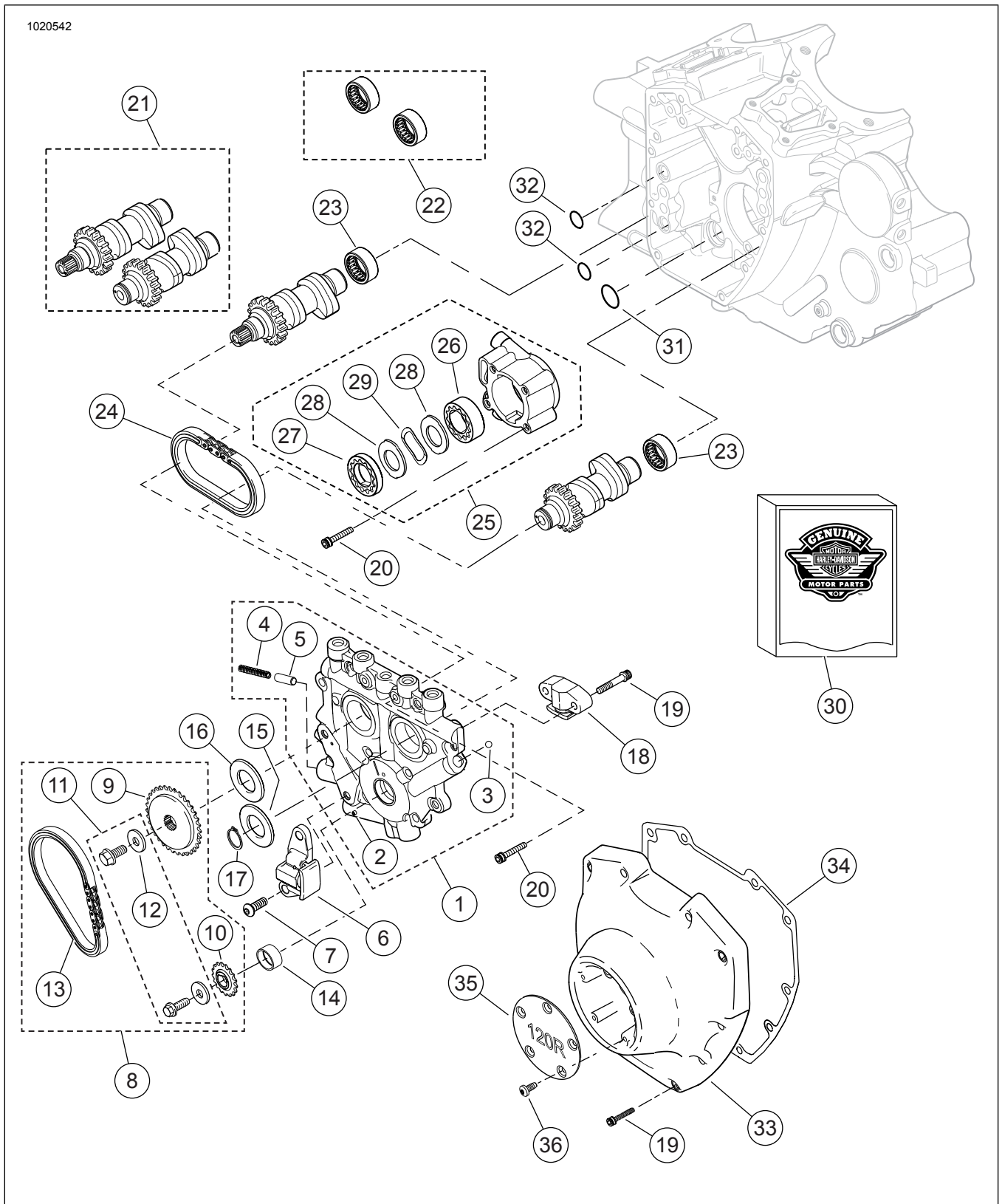
Obrázok 13. Váčkové hriadeľa a kryt váčkového hriadeľa motora Crate SE120R Screamin' Eagle Pro (Alpha)
