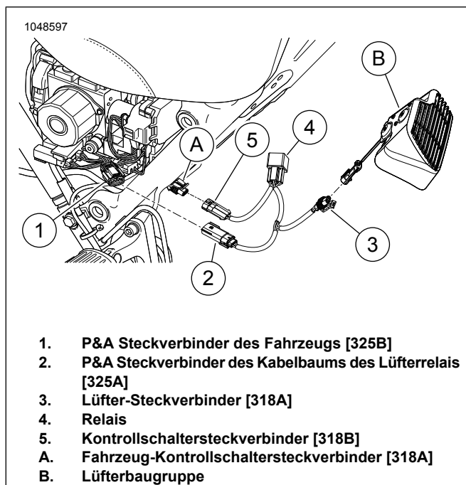
Abbildung 4. Kabelbaumsteckverbinder
