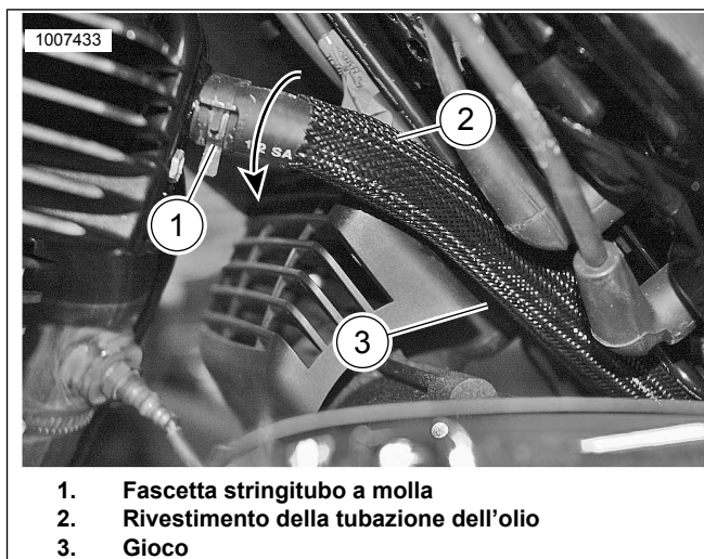
Figura 3. Rivestimento della tubazione posteriore dell'olio
