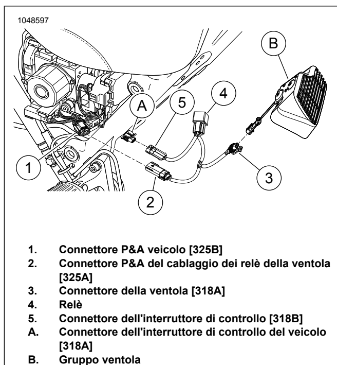
Figura 4. Connettori del cablaggio
