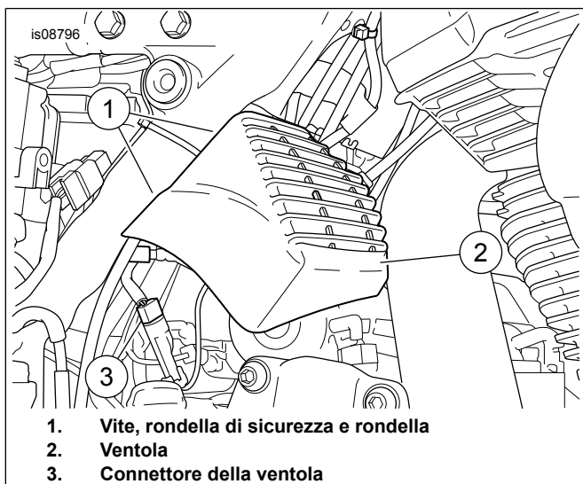
Figura 2. Posizionare la ventola.
