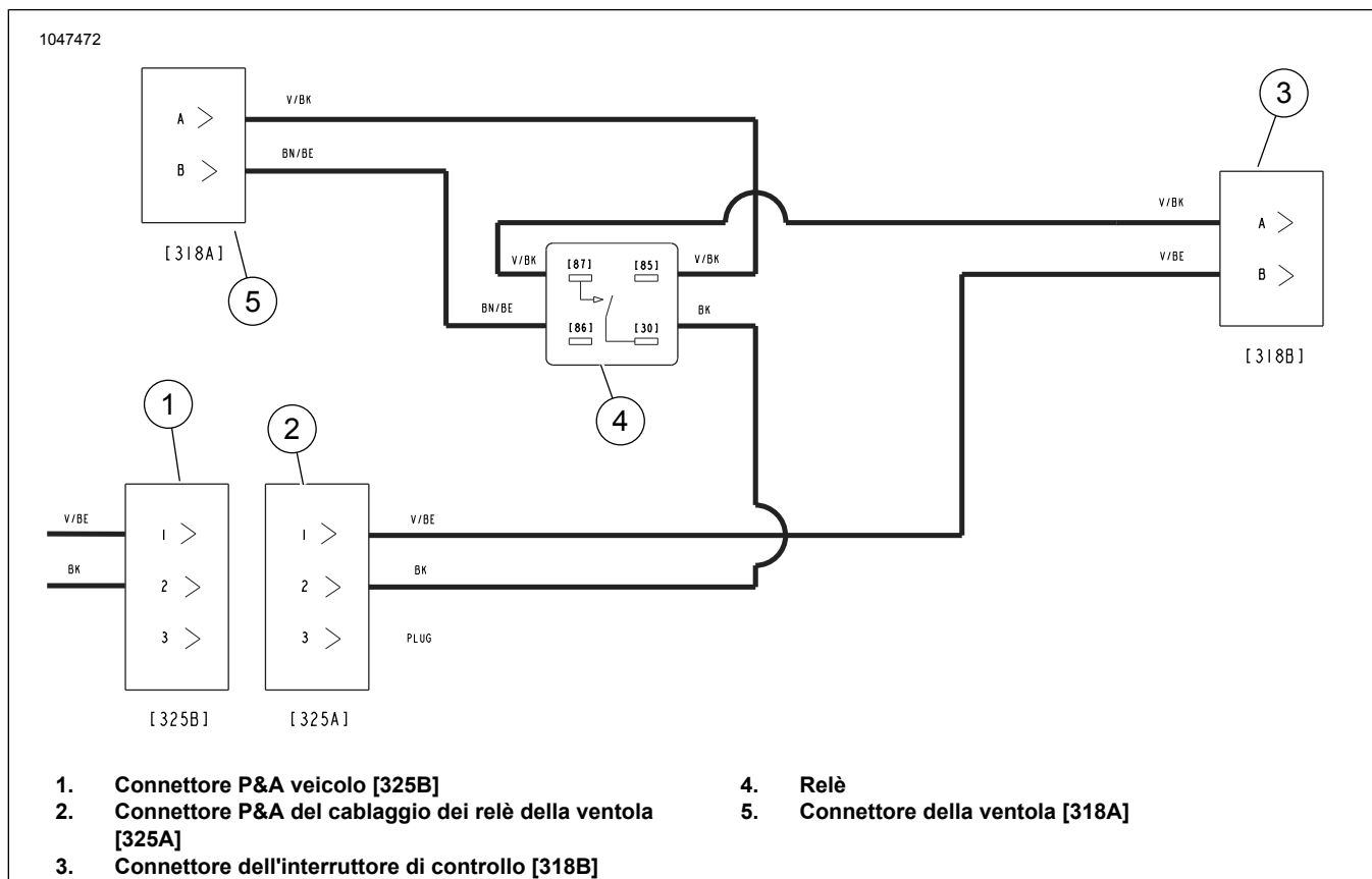
Figura 5. Diagramma del cablaggio della ventola di comfort termico
