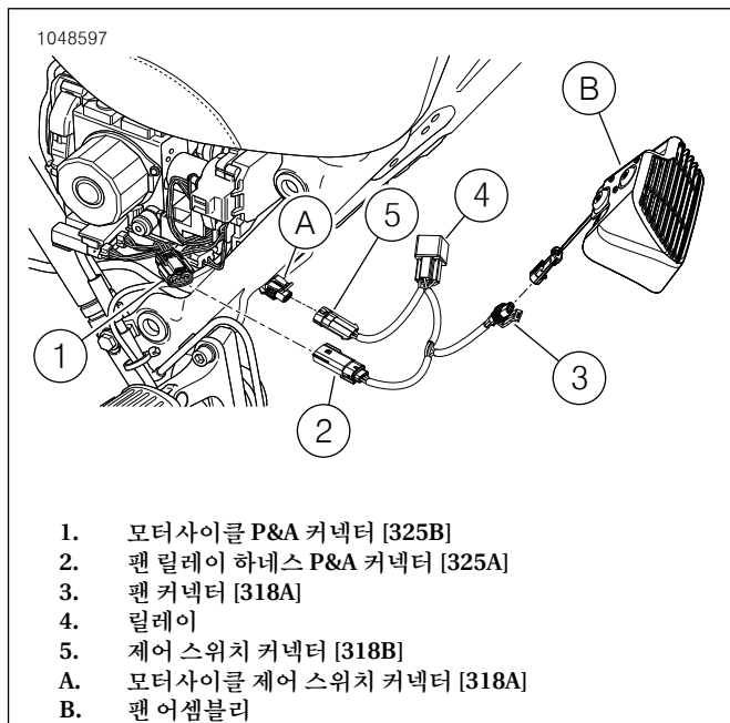
그림 4. 하네스 커넥터
