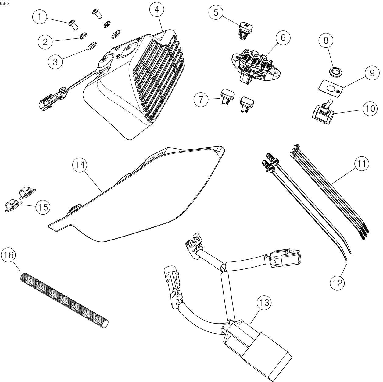
그림 7. 정비 부품: 팬 키트
