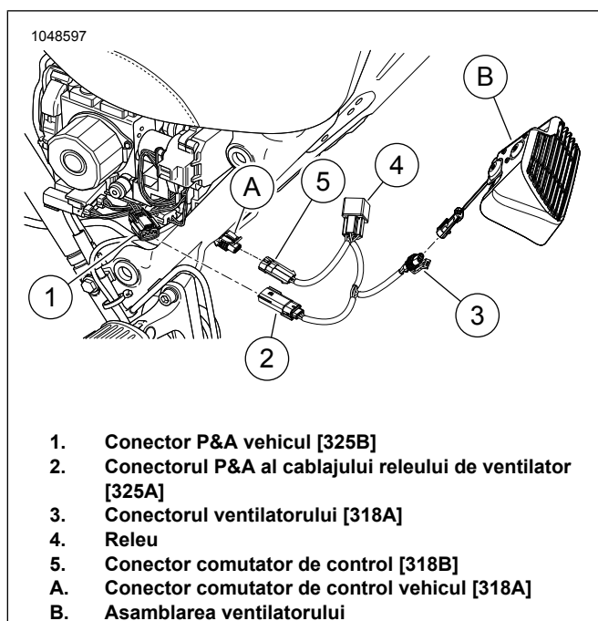
Figura 4. Conectori cablaj
