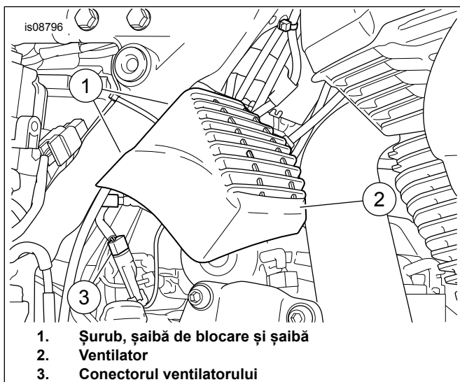
Figura 2. Poziționați ventilatorul
