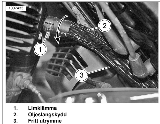
Figur 3. Bakre oljeslangskydd
