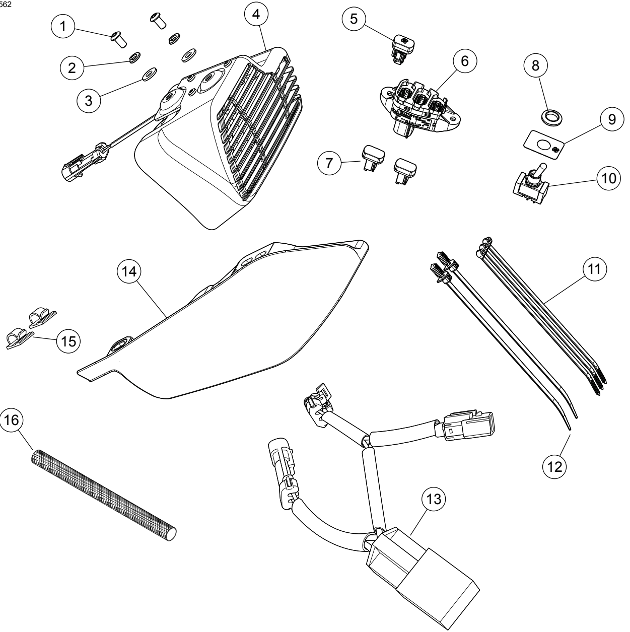
Şekil 7. Servis Parçaları: Fan Kiti
