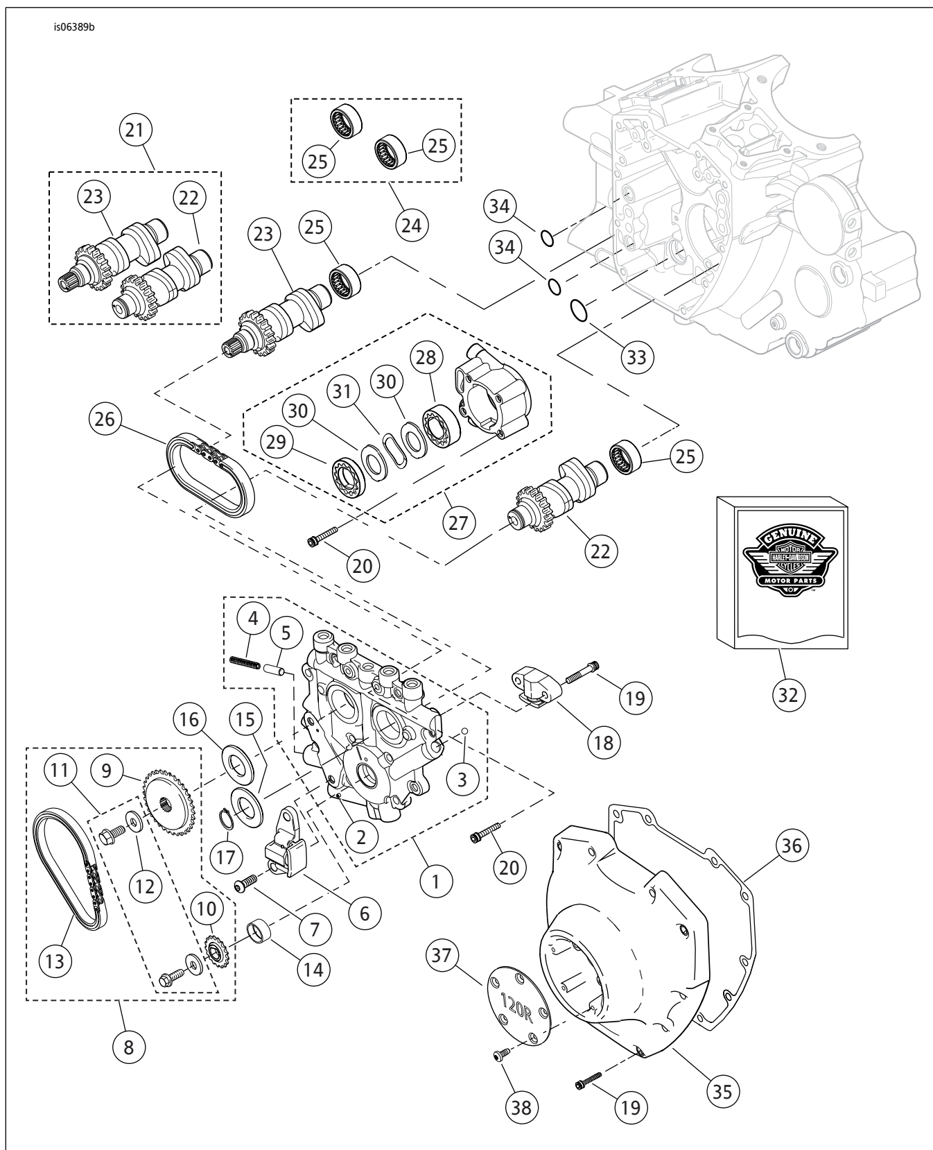
图14。SE120RScreamin' EaglePro箱式发动机( 贝塔 )凸轮轴与凸轮轴罩
