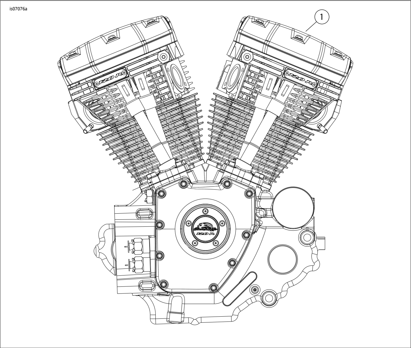
图7。发动机组件：Screamin' EaglePro120R箱式发动机( 贝塔 )总成
