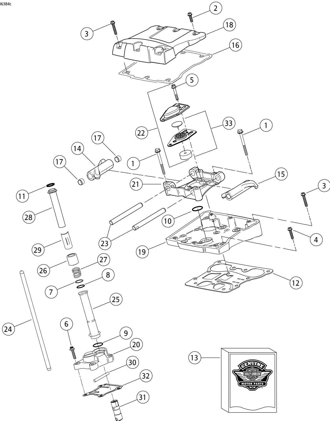
图10。SE120R Screamin' Eagle Pro 箱式发动机(贝塔)摇臂与推杆
