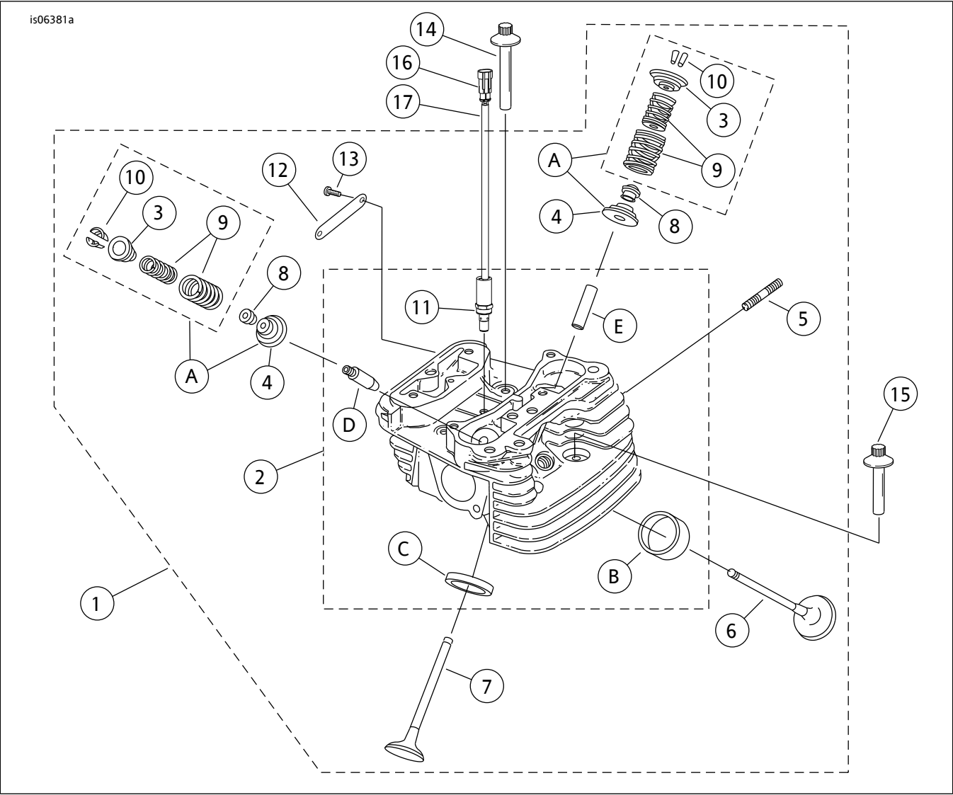
图9。SE120RScreamin' EaglePro箱式发动机( 贝塔 )汽缸头与气门
