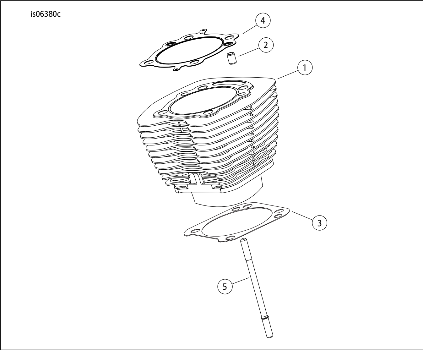
图8。SE120RScreamin' EaglePro箱式发动机( 贝塔 )汽缸
