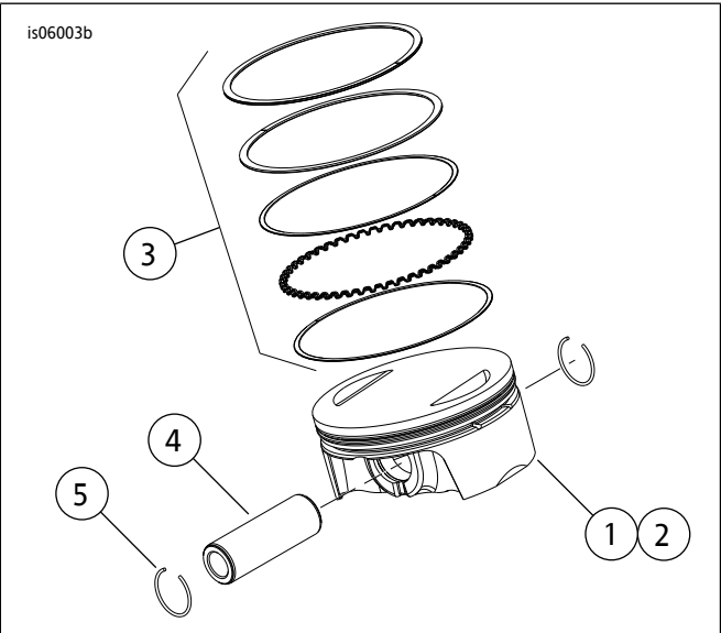
图5。活塞组件
