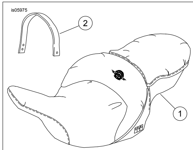
Afbeelding 7. Serviceonderdelen: Road Zeppelin zadel
