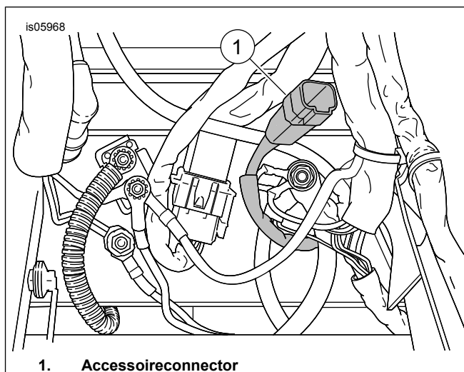
Afbeelding 2. Locatie accessoireconnector (onder het zadel)
