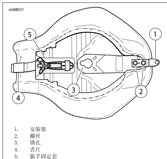
图1。支架、螺丝、锁孔和舌片
