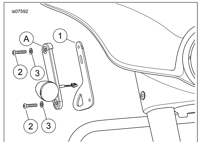
Figura 1. Installazione della staffa di ancoraggio
