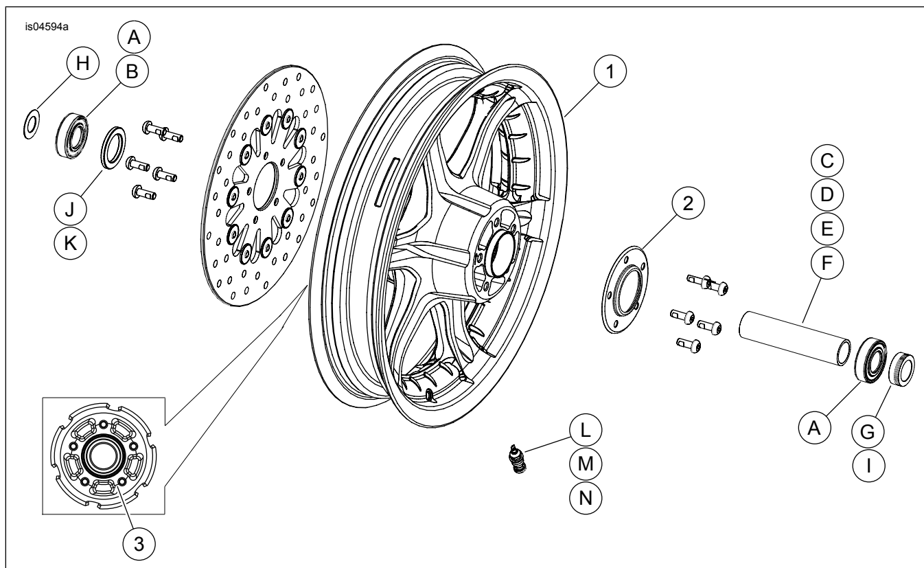
Afbeelding 2. Serviceonderdelen: 6-Spaaks voorwiel met sleuven (16 inch wiel afgebeeld)
