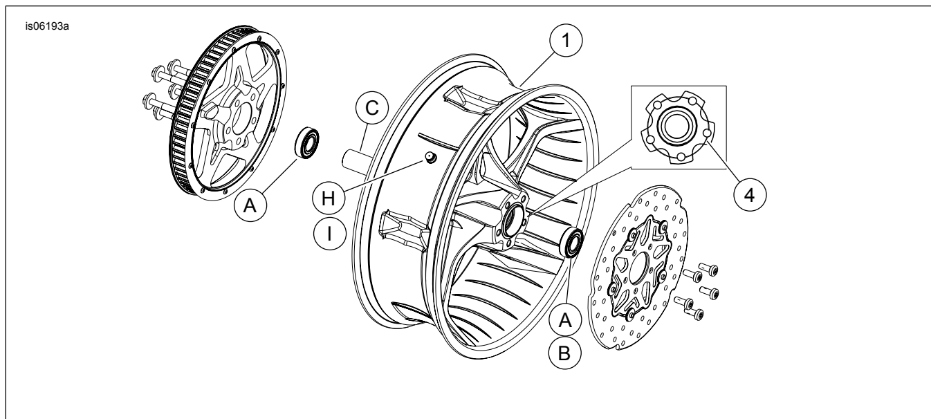
Afbeelding 1. Serviceonderdelen: Stinger achterwiel
