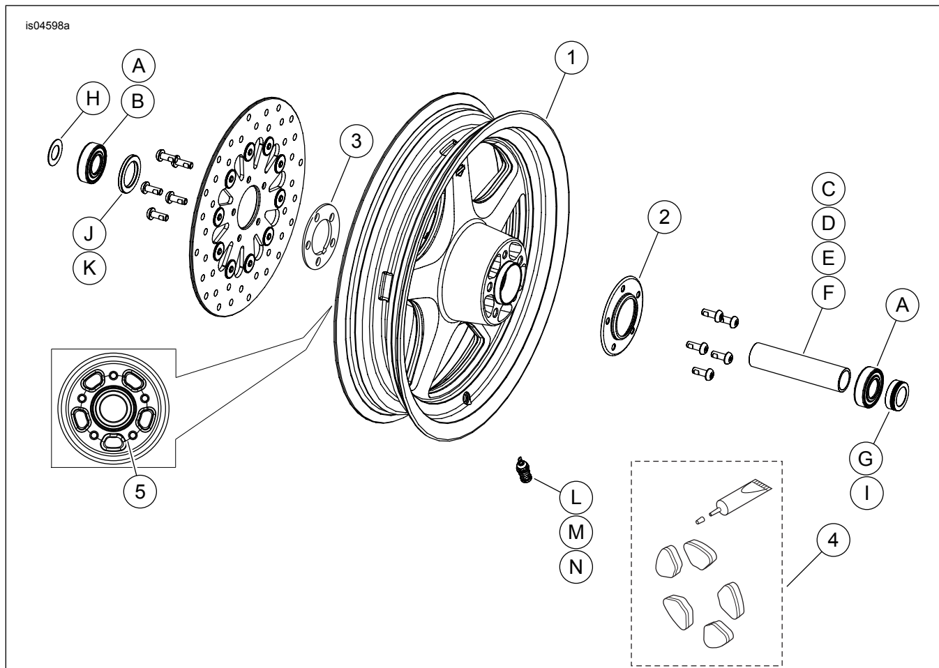
Afbeelding 2. Serviceonderdelen: THUNDERSTAR VOORWIELSETS (16 inch wiel afgebeeld)
