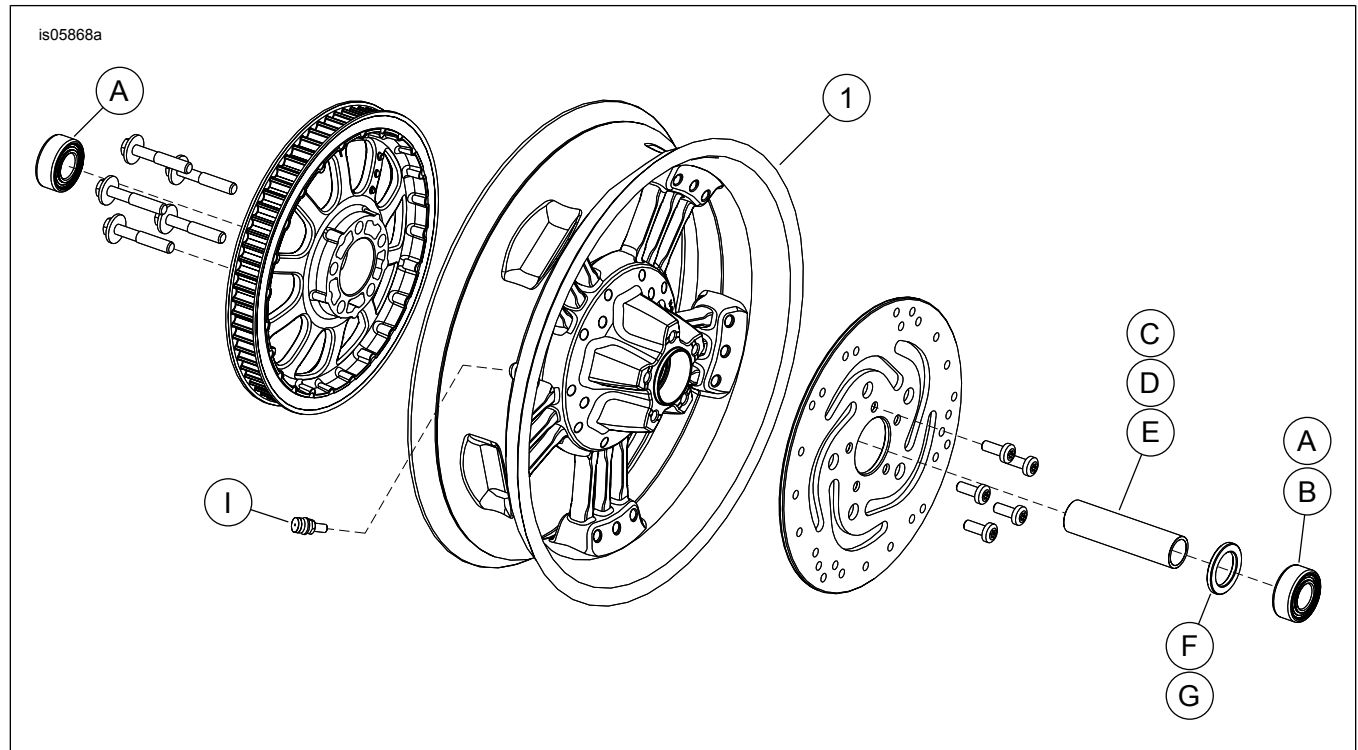
Afbeelding 1. Serviceonderdelen: Magnum 5-achterwiel (17 inch wiel afgebeeld)
