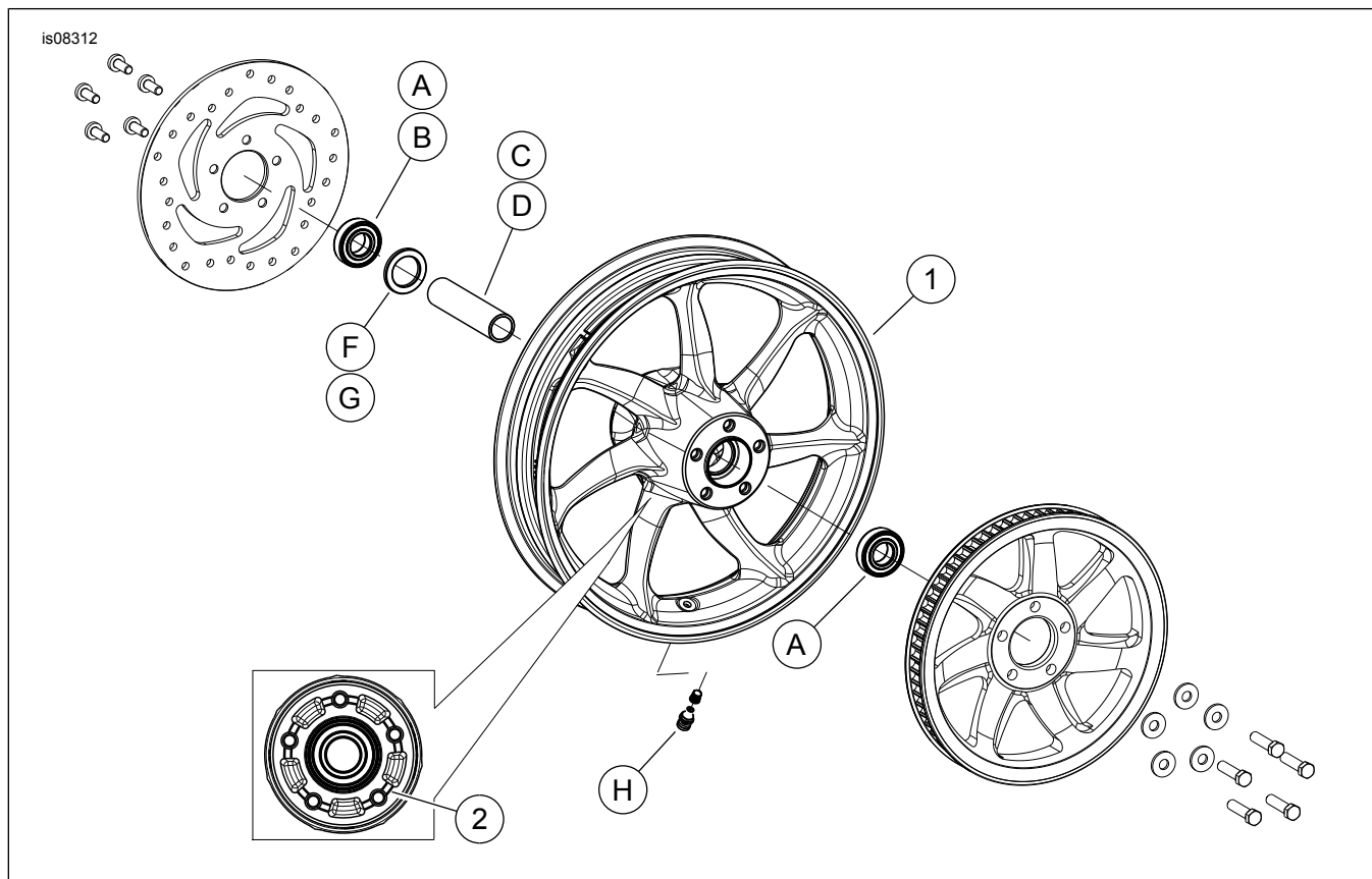
Afbeelding 1. Serviceonderdelen: Machete-achterwielen (16 inch afgebeeld)
