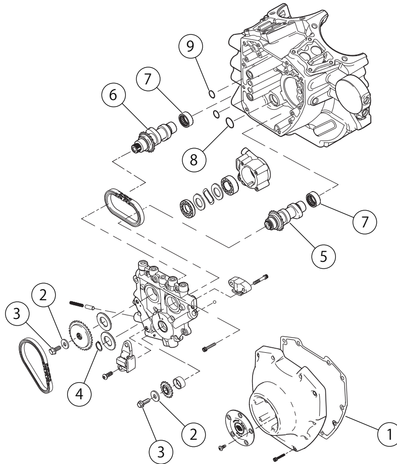
図3。交換用パーツ:Screamin' EaglePROTC103 (1690cc) ステージ4キット
