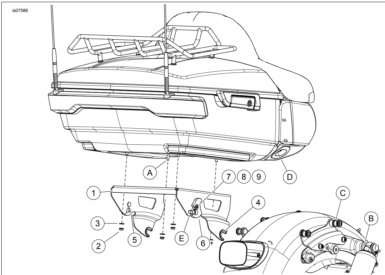
is07586 Figura 2. Parti di ricambi, portabagagli Tour-Pak per sella monoposto rimovibile
