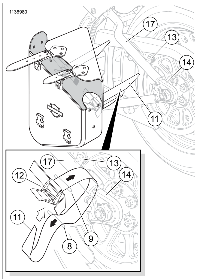
Figure 9. Ikabit ang Likurang Strap - 2018 na Softail at mas bago
