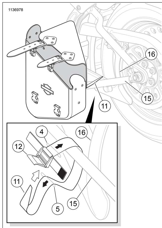
Figure 7. Ikabit ang Pang-ibabang Strap - 2018 na Softail at mas bago
