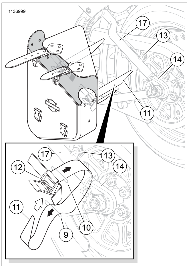
Figure 5. Ikabit ang Likurang Strap - 2017 na Softail at mas luma
