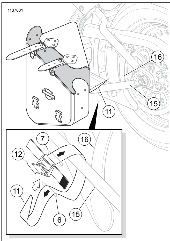
Figure 3. Ikabit ang Pang-ibabang Strap - 2017 na Softail at mas luma
