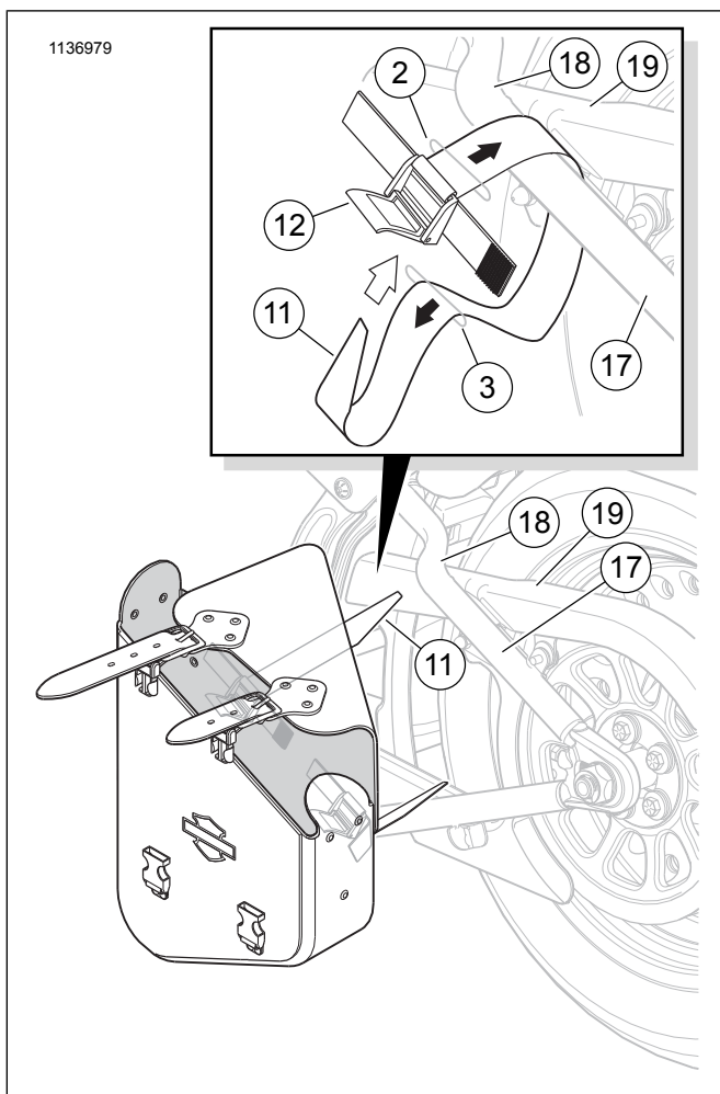
Figure 8. Ikabit ang Harapang Strap - 2018 na Softail at mas bago
