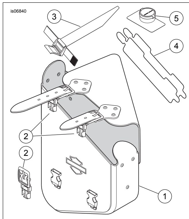
Figure 10. Mga Pamalit na Piyesa: Swingarm Bag ng Softail
