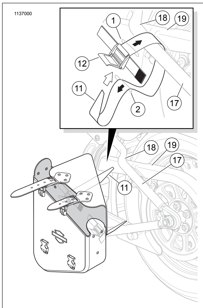
Figure 4. Ikabit ang Harapang Strap - 2017 na Softail at mas luma
