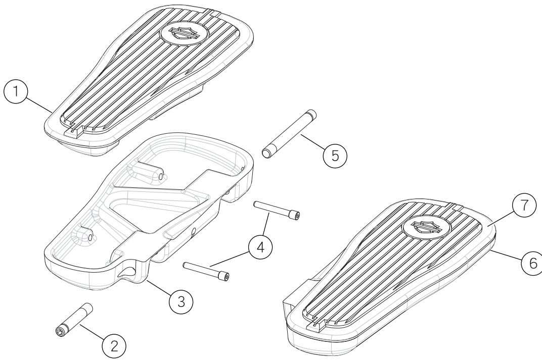
圖2。維修零件乘客腳踏板工具包
