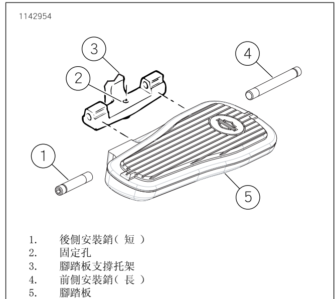
圖1。腳踏板支架和腳墊
