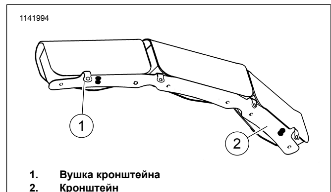
Малюнок 1. Низ сумки на обтічник
