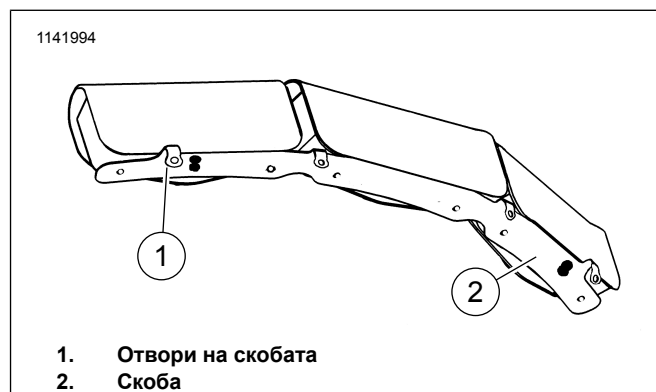
Фигура 1. Дъно на чантата за обтекател
